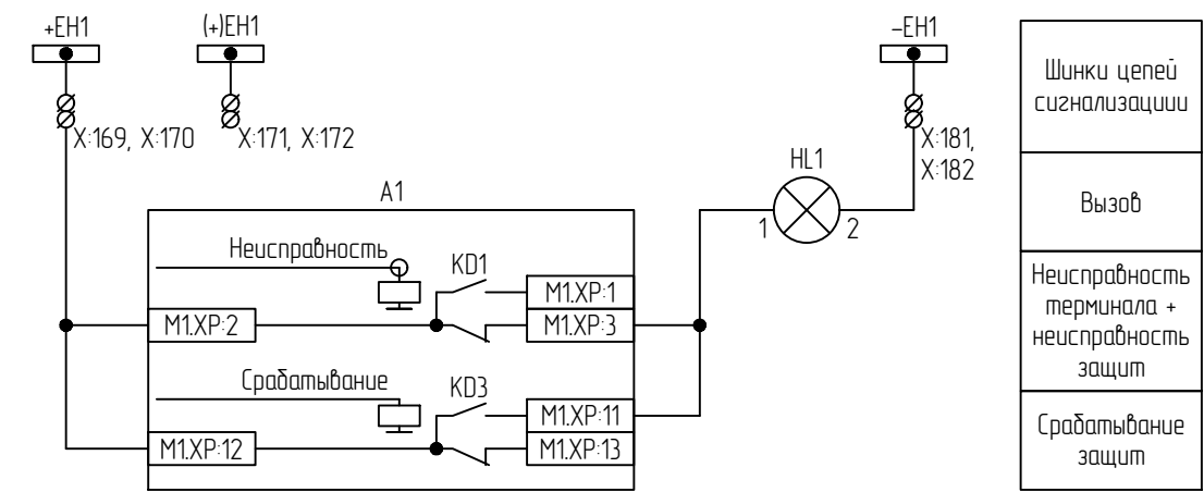
Цепи РАС
